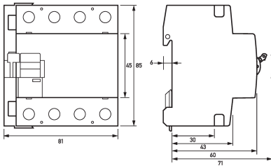
Maßzeichnung Gruppenansicht
