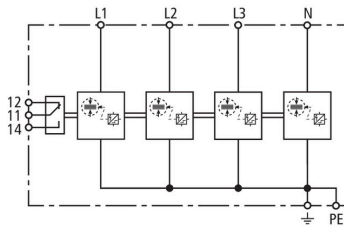
Prinzipialschaltbild DSH TNS 255 FM
