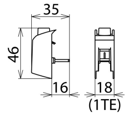
Maßbild STAK 25
