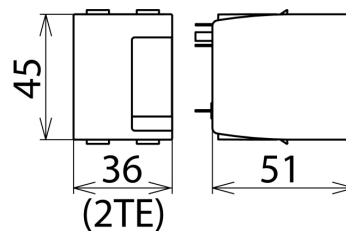
Maßbild DR MOD 4P 255
