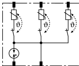
Prinzipialschaltbild DR MOD 4P 255
