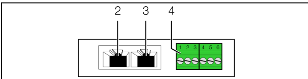
Abb. 9: Rückseite des Universalsensors
