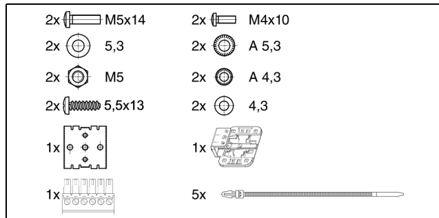
Abb. 1: Beigelegtes Zubehör
