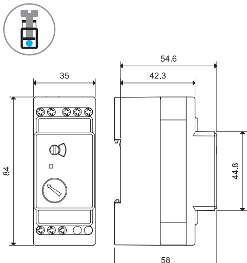
Typ 72.01/11 Schraubklemmen
