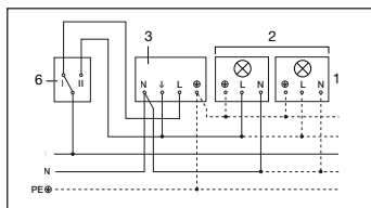
4. Tilkopling via vendedbryter for permanent belysning og automatisk drift Posisjon I: automatisk drift Posisjon II: manuell drift permanent belysning
