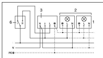
4. Koppling via 2-polig brytare för fast sken respektive automatisk
