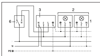
4. Pieslēgums ar maiņas slēdzi ilgstošā apgaismojuma un automātikas režīmam Pozīcija I – automātikas režīms Pozīcija II – ilgstošā apgaismojuma manuālais režīms Uzmanību! Iekārtu izslēgt nav iespējams, iespējama ir tikai izvēle starp pozīciju I un pozīciju II.
