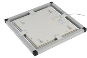
Rückseite Heizelement
