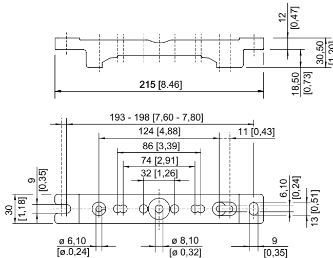
Montageschiene
