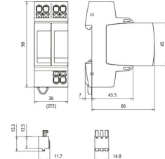
Maßbild DG MP TT 2P 275 FM
