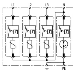
Principalschaltbild DG M TT 320
