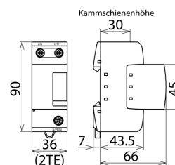
Maßbild DB M 1 150
