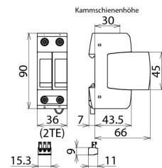
Maßbild DG M TT 2P 320 FM
