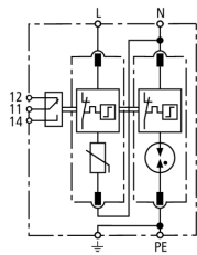
Prinzipschaltbild DG M TT 2P 320 FM
