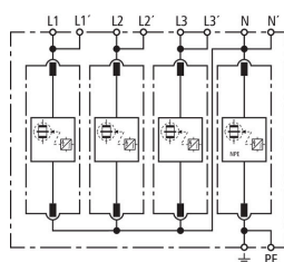
Principalschaltbild DV M TT 255
