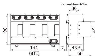
Maßbild DV M TT 255
