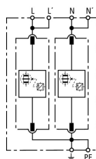
Principalschaltbild DV M TN 255
