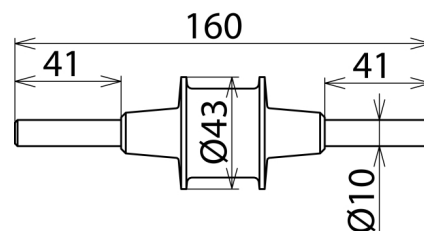
Maßbild TFS
