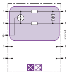
Prinzip Schaltbild BXT ML2 BD 180
