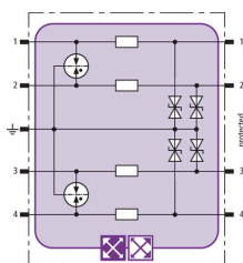
Prinzipialschaltbild BXT ML4 BE 5
