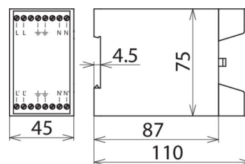
Maßbild NF 10
