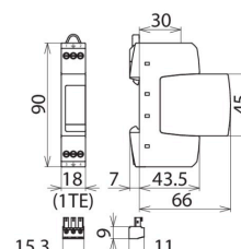
Maßbild DR M 2P 75 FM
