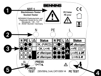
Kuva 1: Laitteen etupuoli
