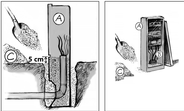
A-prázdne teleso B-tesniaca zátka C-suchý biely piesok
