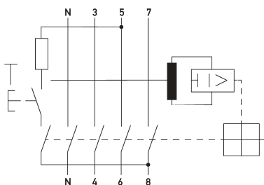
Anschlussschema
