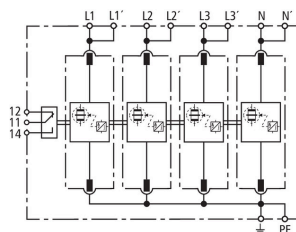
Prinzip Schaltbild DV M TNS 255 FM
