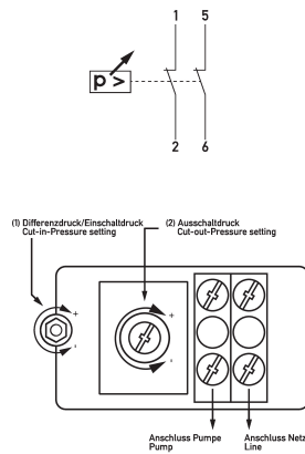
Anschlussschema
