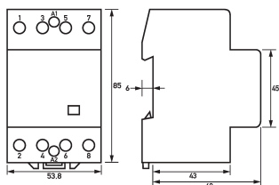
Maßzeichnung Gruppenansicht
