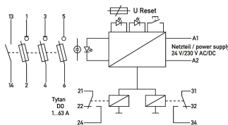
Anschlussschema
