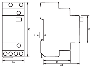
Maßzeichnung Gruppenansicht
