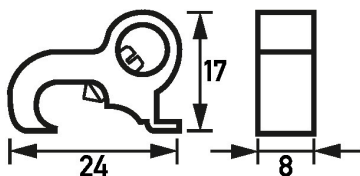
Maßzeichnung Gruppenansicht
