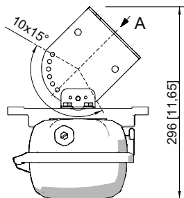
Montagebügel montiert in Montageschiene
