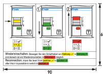
Maßzeichnung Gruppenansicht
