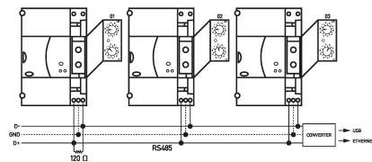
Anschlusschema
