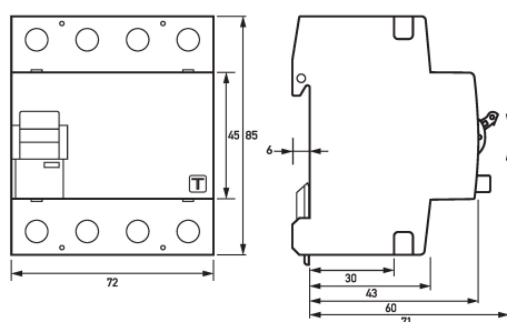
Maßzeichnung Fehlerstromschutzschalter DFS 4 040-4/0,30-A
