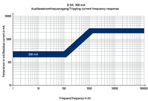
Diagramme Fehlerstromschutzschalter DFS 4 125-4/0,30-B SK
