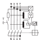
Schaltungsbeispiel Fehlerstromschutzschalter DFS 4 040-4/0,03-A EV
