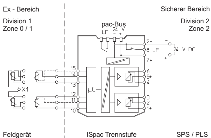
Anschlussplan 9180/2.-77-11
