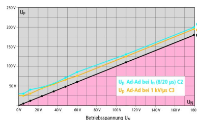
Schutzpegeldiagramm DBX U4 KT BD S 0-180
