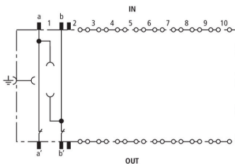
Prinzipialschaltbild BM 10 DRL
