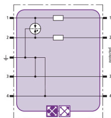
Principalschaltbild BXT ML2 B 180
