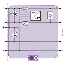
Principalschaltbild BXTU ML2 BD S 0-180
