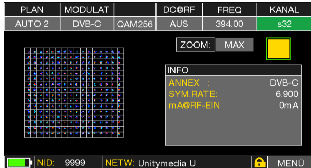
256 QAM Konstellation
