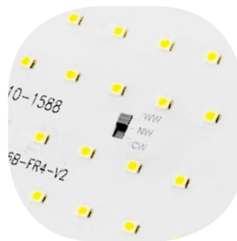
Lichtfarbe in 3000K Warmweiß / 4000K Neutralweiß / 5700K Tageslichtweiß durch DIP-Schalter einstellbar
