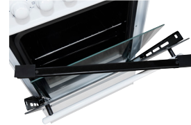
Glasscheibe herausnehmbar Einfaches herausnehmen der Ofentür-Glasscheibe.
