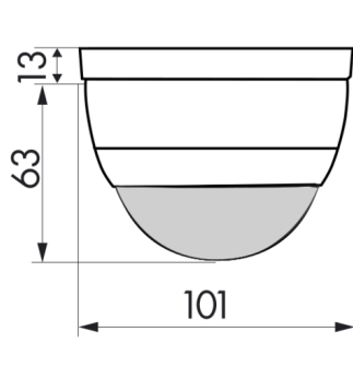
Bemaßung 92140
