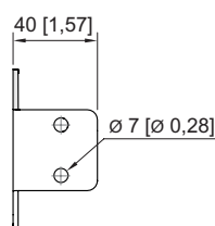
Montageklammer Fläche
