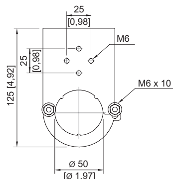
Montageklammer Fläche
