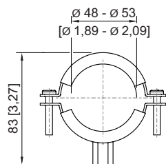
Montageklammer Gewinde
