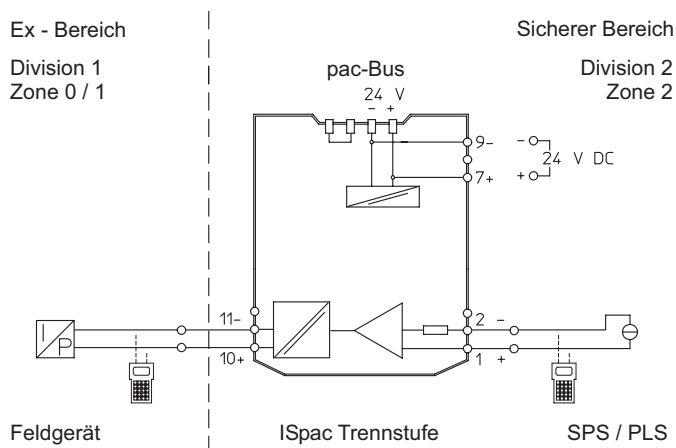
Anschlussplan 9165/16-11-10
