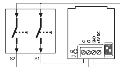
Anschluss Taster
