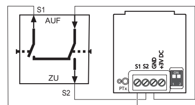
Anschluss Jalousieschalter
