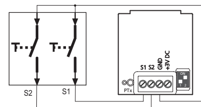
Anschluss Schalter
