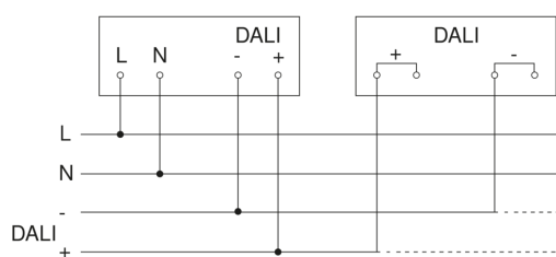
Schaltplan Vernetzung DALI-2 APC mit DALI-2 IPD
