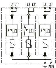
Prinzipschaltbild DG MP TNC 275 FM
