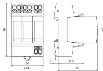
Maßbild DG MP TNC 275 FM
